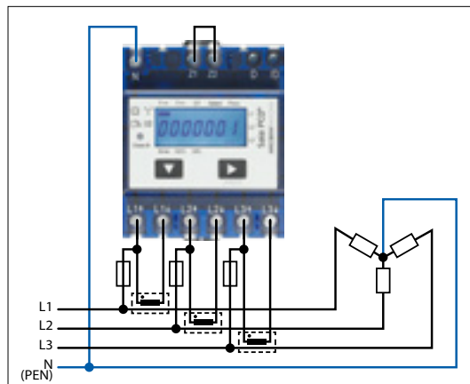
▲ Angeschlossener Wandlerenergiezähler
