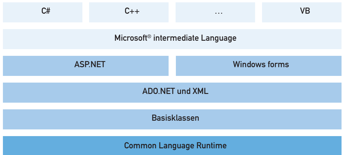
Microsoft®.NET-Struktur
