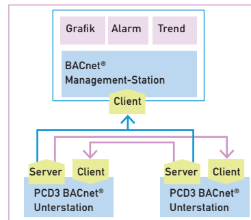
BACnet® Client / Server Funktionalität in der Automationsstation Saia®PCD3
