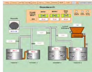
Schematische Darstellung von 4 Fermentern mit Rührwerken, Gasspeicher und Feststoffeinbringung über ein Schneckenwerk.
