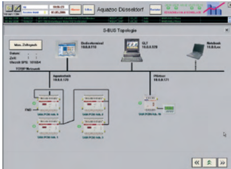
S-Bus Topologie, dargestellt auf dem Touch-Panel
