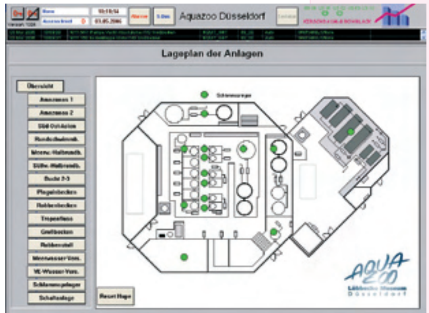
Lageplan der Anlage Aquazoo, dargestellt auf dem Touch-Panel
