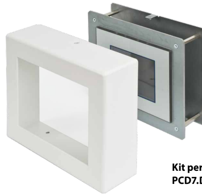
Kit per il montaggio incassato PCD7.D457-IWS2
