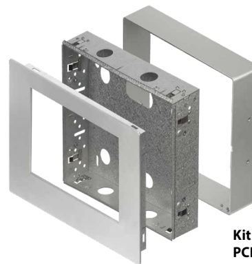
Kit per il montaggio su parete PCD7.D457-OWS1
