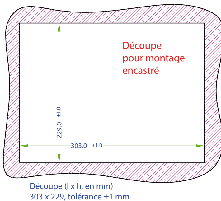
Découpe frontale pour montage encastré
