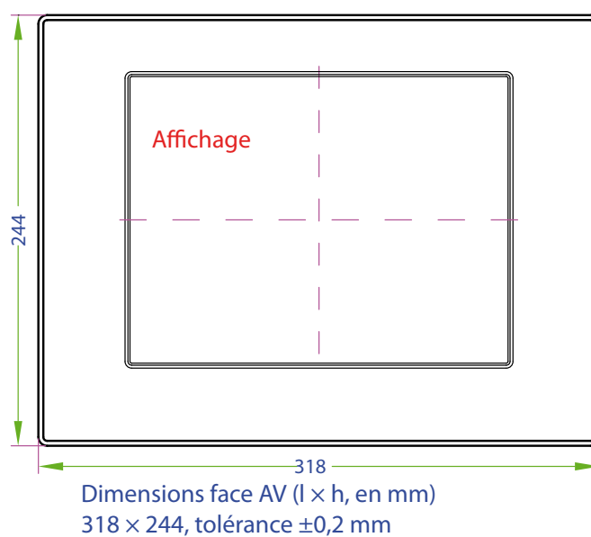
Vue de face de la face AV
