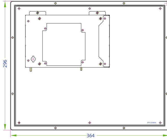
Blick auf die Geräterückseite
