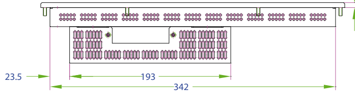
Blick auf die Geräteoberseite
