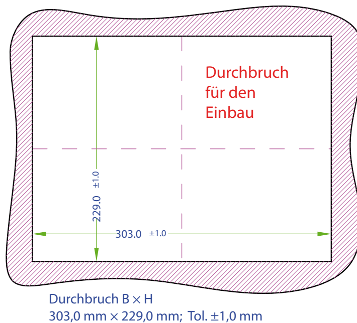
Fronttafeldurchbruch für den Einbau
