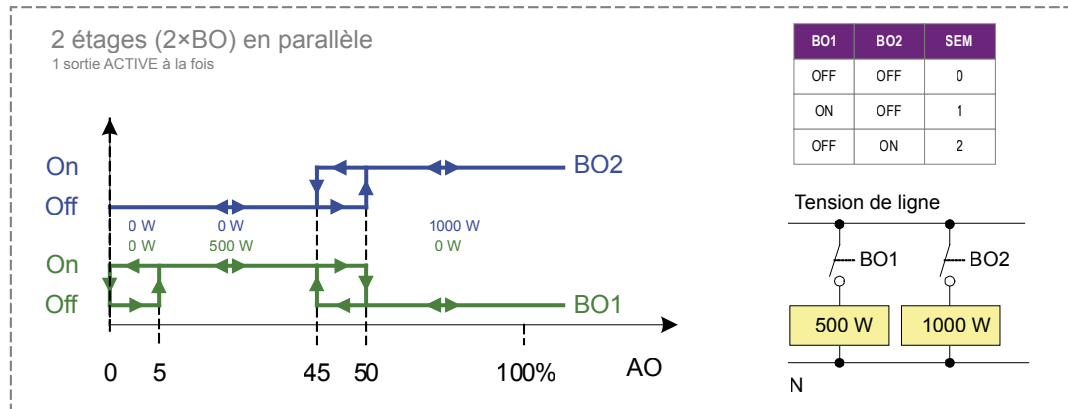
Image 28. Sortie libre : 2 vitesses, 2×BO en parallèle
