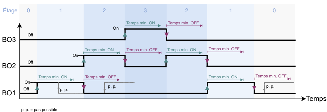
Image 33. Sortie à 3 vitesses : comportement de commutation et temporisation minimale avant activation/désactivation
