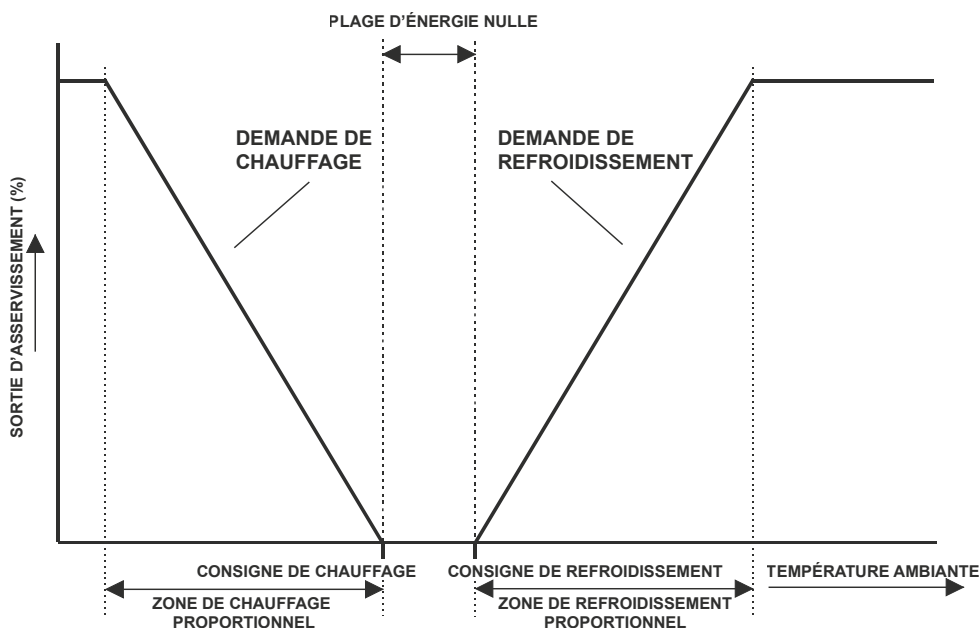
Image 22. Schéma représentant la séquence de régulation (exemple d'une régulation P)
