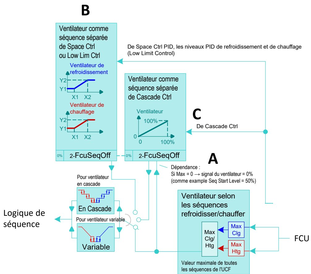
Image 24. Stratégie de contrôle du ventilateur
