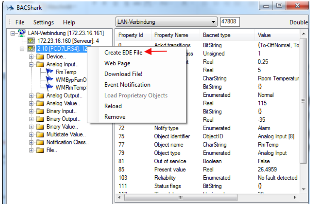
Image 2. Création de fichiers .EDE
