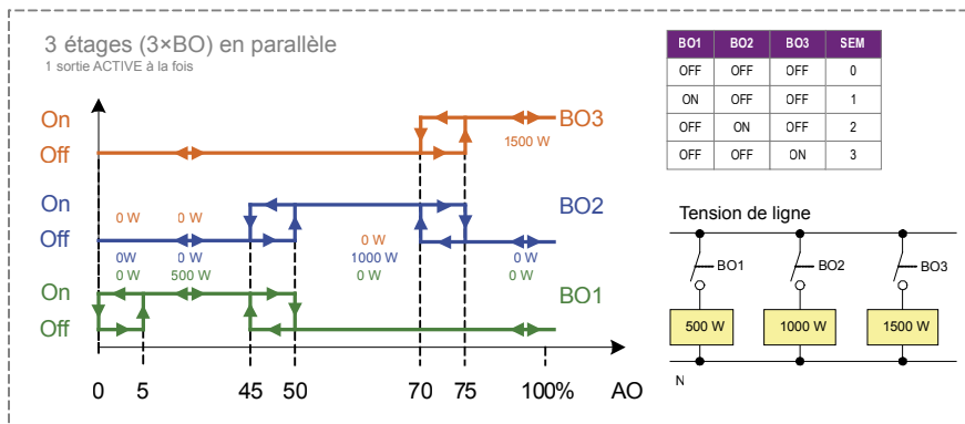
Image 31. Sortie libre : 3 vitesses, 3×BO en parallèle
