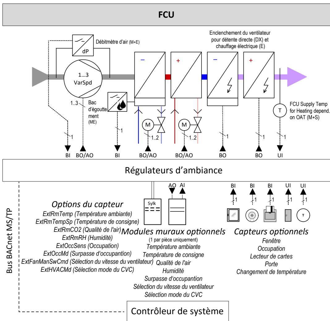
Image 10. Application de régulation par ventilo-convecteur
