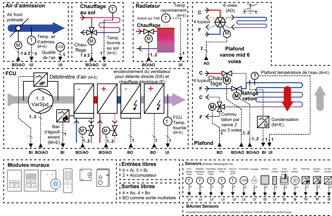
Image 9. Vue d'ensemble des applications
