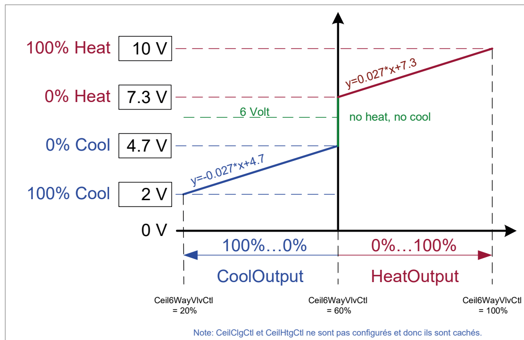
Fig. 35. Fonctionnement du capteur de température pour basculement chauffage / refroidissement
