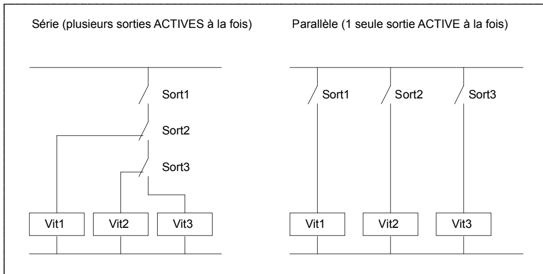
Image 24. Câblage d'un ventilateur à vitesses multiples
