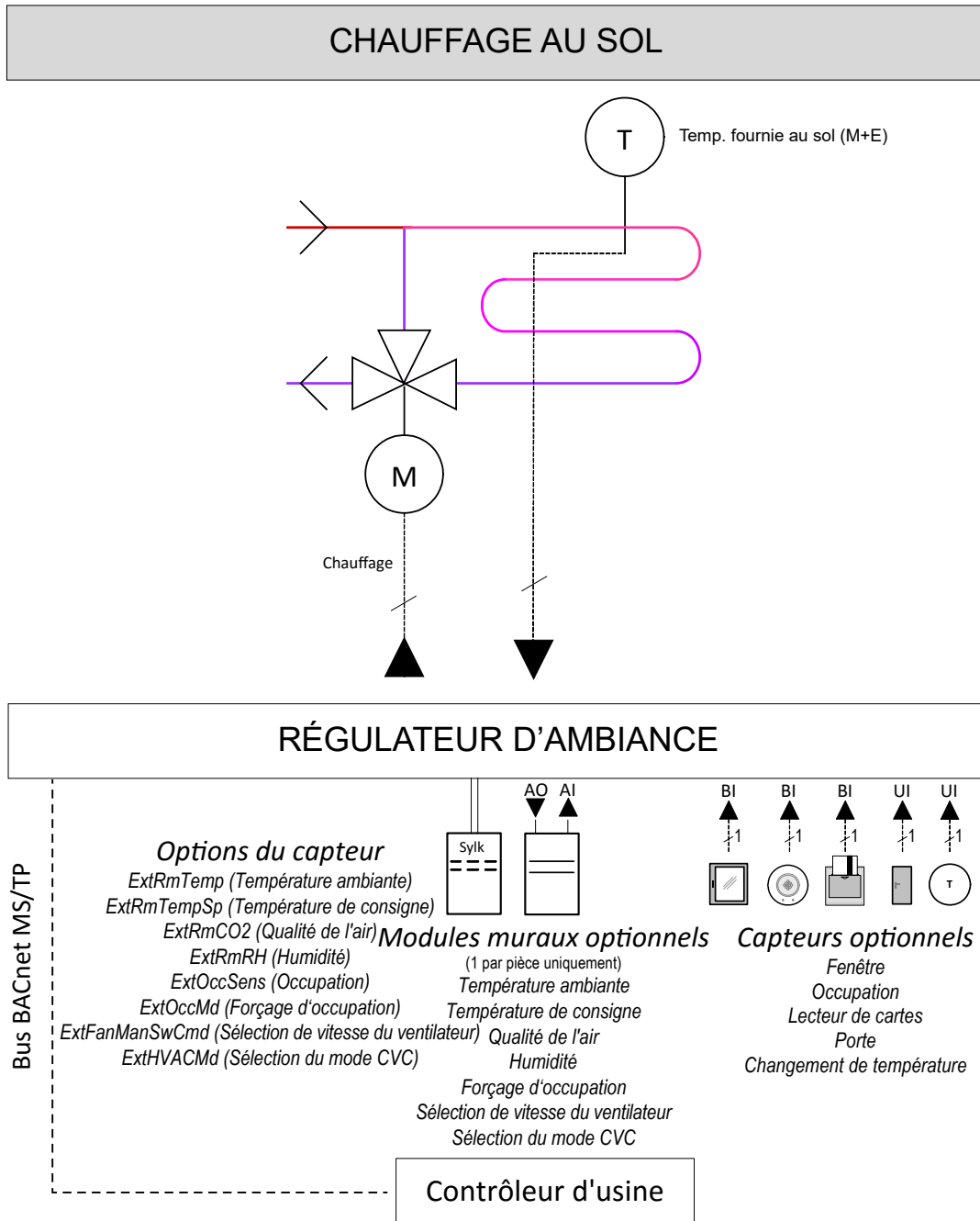
Image 16. Application de régulation par chauffage au sol
