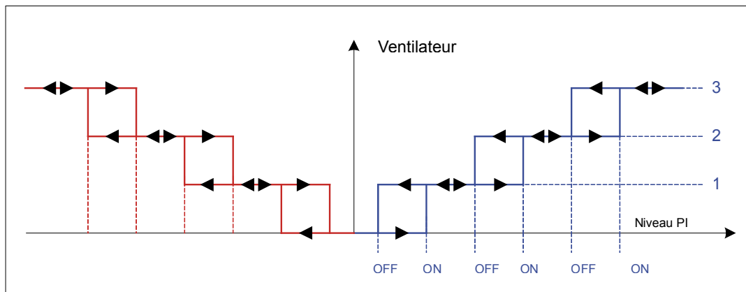
Image 25. Commutation d'un ventilateur à vitesses multiples selon la demande de régulation
