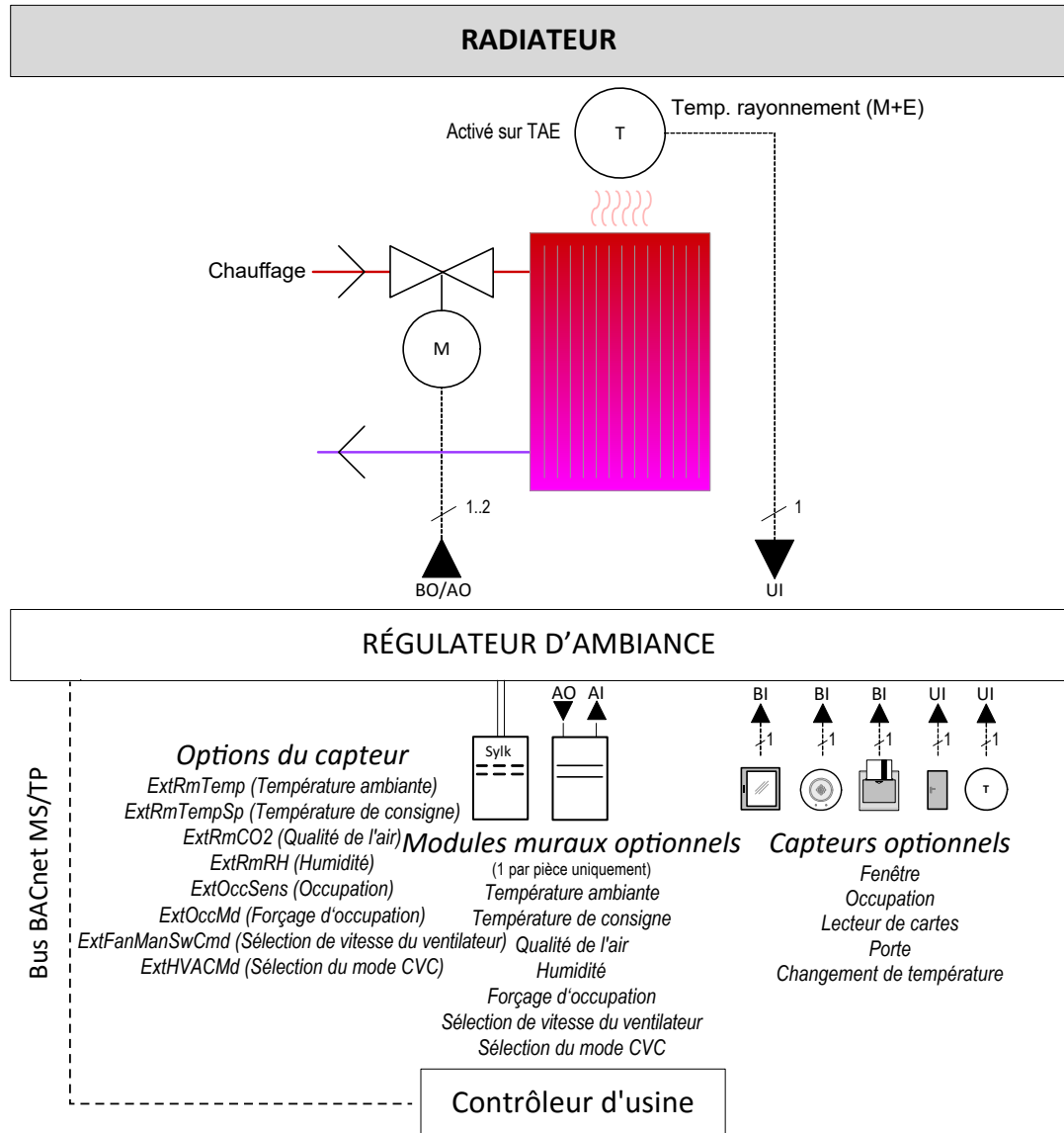
Image 15. Application de régulation par radiateur
