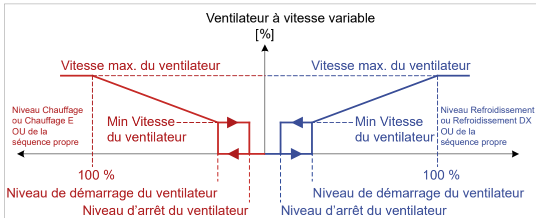
Image 27. Vitesse d'un ventilateur à vitesse variable selon la demande de régulation
