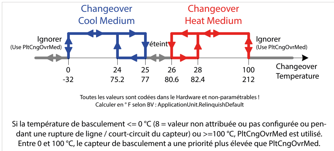
Fig. 34. Fonctionnement du capteur de température pour basculement chauffage / refroidissement
