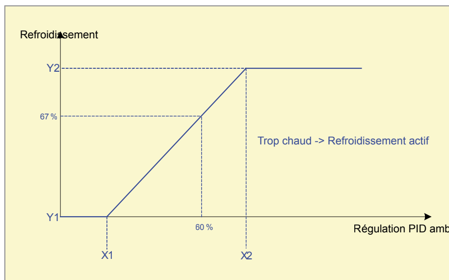
Image 23. Configuration d'une séquence (exemple d'un refroidissement VC)
