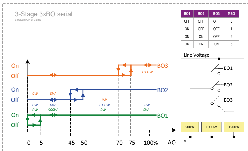
Image 32. Sortie libre : 3 vitesses, 3×BO en série
