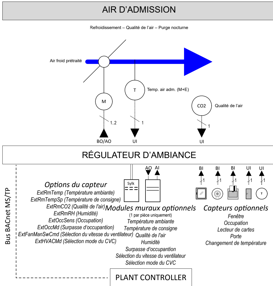
Image 17. Application de régulation par air d'admission
