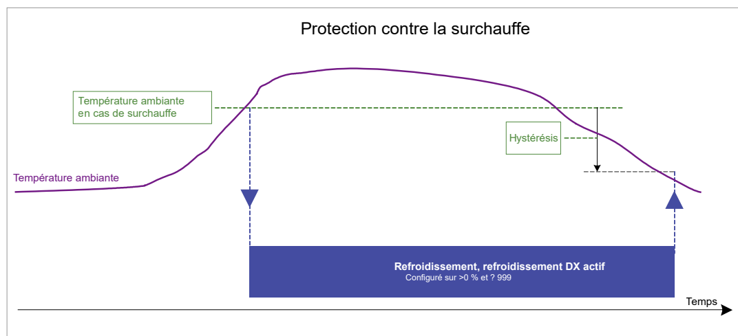
Image 19. Exemple de protection contre la surchauffe
