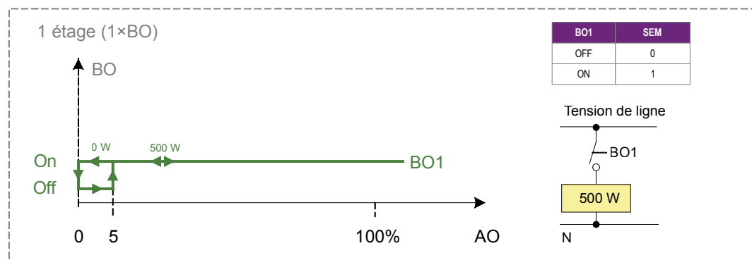
Image 27. Sortie libre : 1 vitesse, 1×BO
