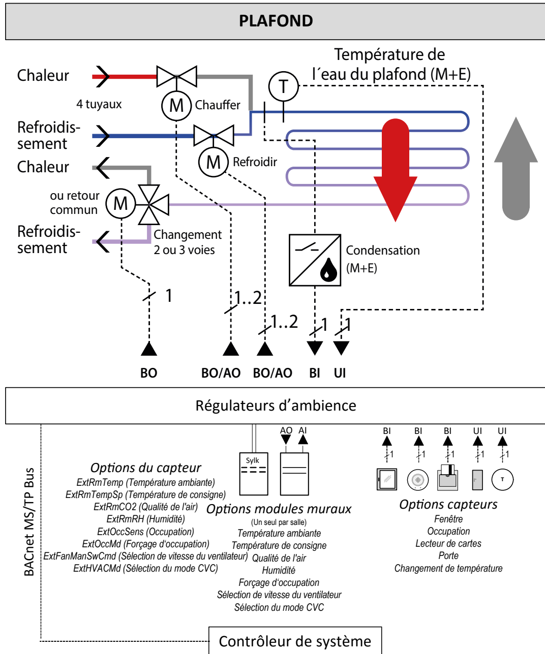
Image 11. Application de régulation par les plafonds
