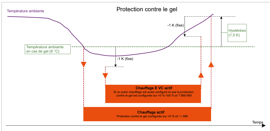
Image 18. Exemple de protection contre le gel
