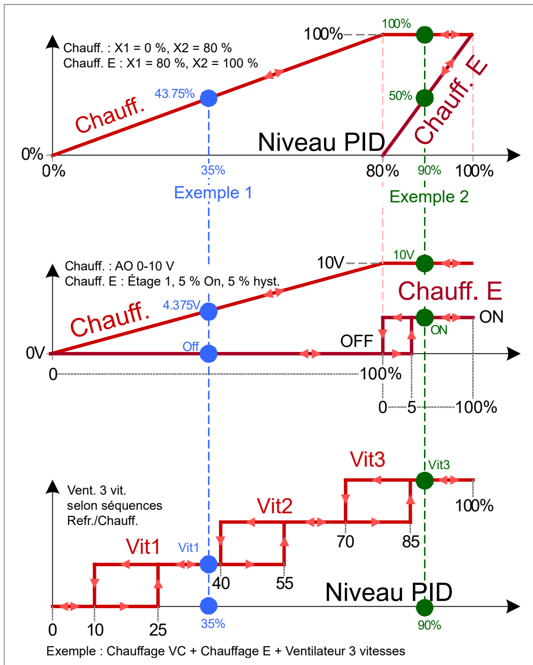
Image 26. Ventilateur à vitesses multiples, exemple de régulation du chauffage et du chauffage électrique
