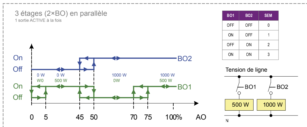
Image 30. Sortie libre : 3 vitesses, 2×BO en parallèle
