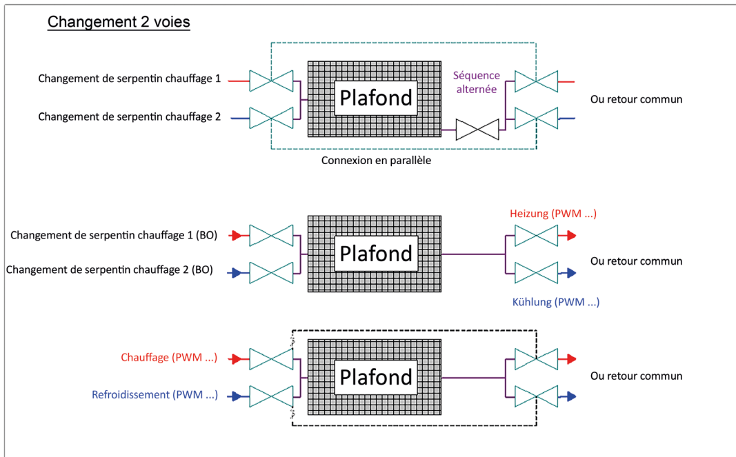
Image 13. Configuration de la commutation du plafond avec une vanne 2 voies
