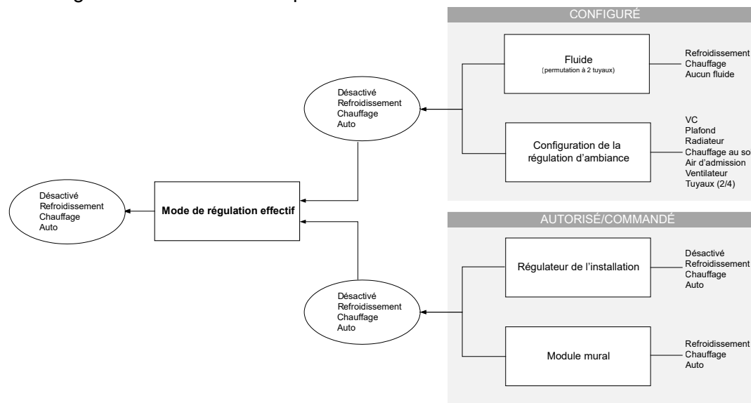
Image 21. Mode de régulation effectif
