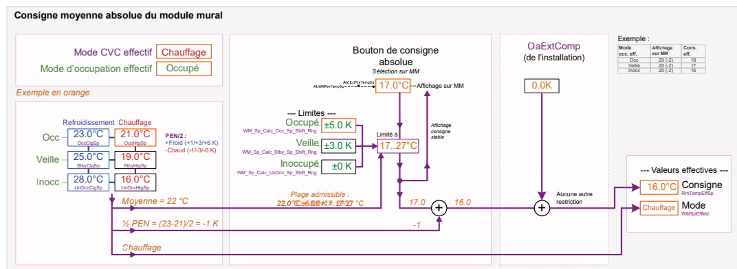
Image 26. Réglage de consigne absolue
