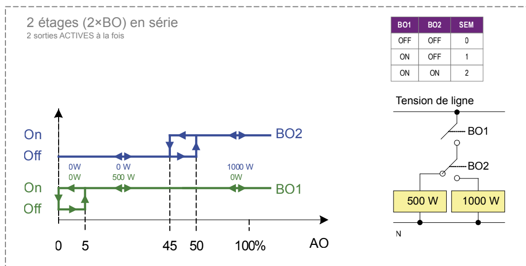
Image 29. Sortie libre : 2 vitesses, 2×BO en série
