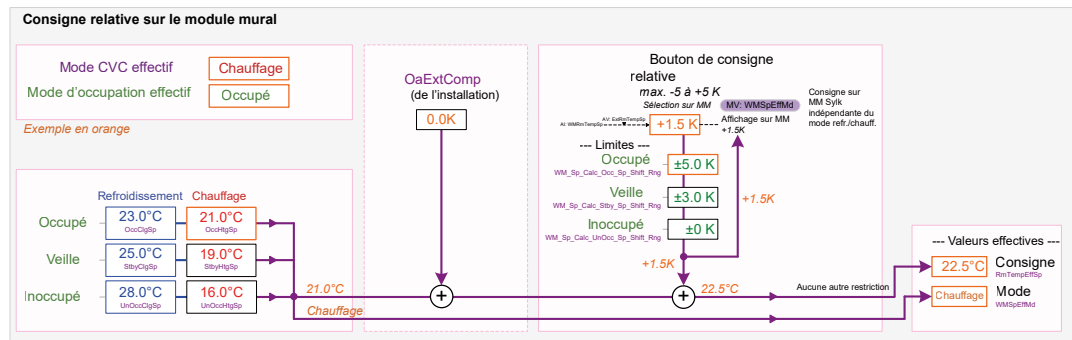
Image 25. Réglage de consigne relative
