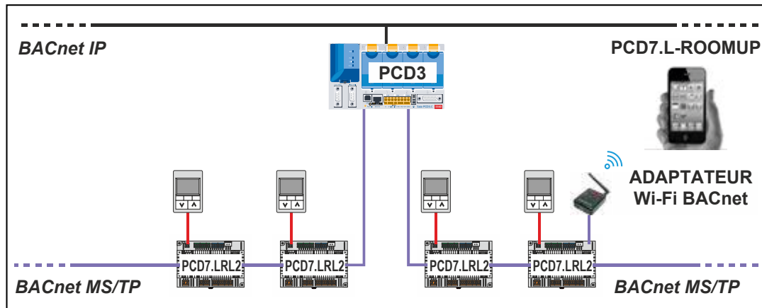
Image 1. Architecture avec un automate PCD3
