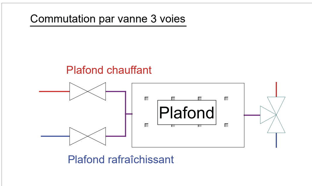
Image 14. Configuration de la commutation du plafond avec une vanne 3 voies
