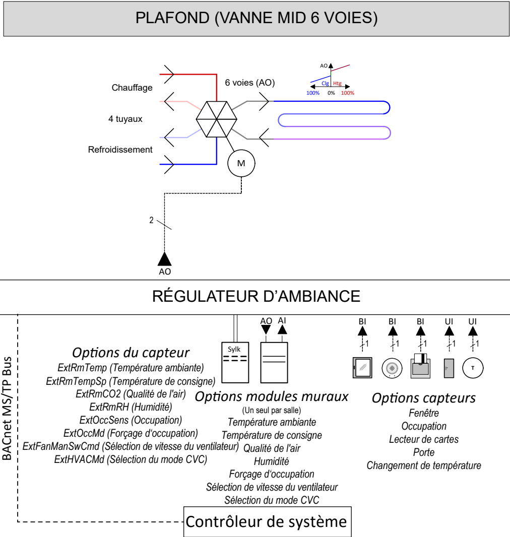
Image 12. Application de régulation des vannes MID 6 voies des plafonds
