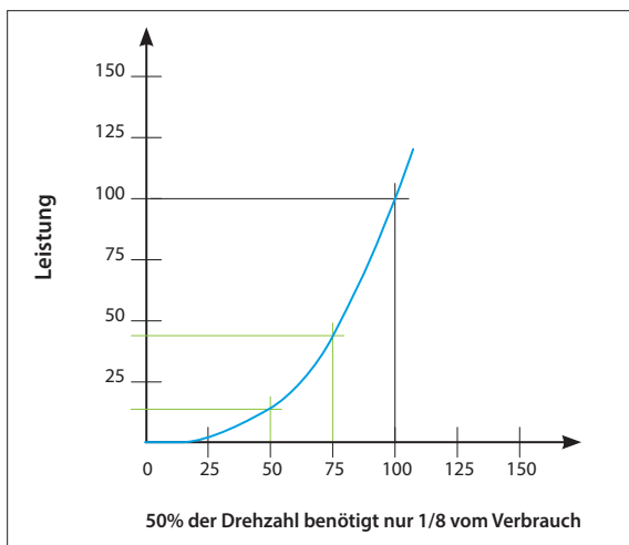
▲ Leistung/Drehzahl-Kurve
