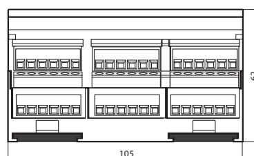
Gehäuse mit 6 TE (105 mm) Passend für Elektroschaltschrank (gemäss DIN 43880, Grösse 2 x 55 mm)
