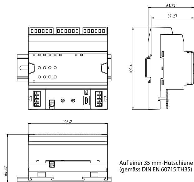
Gehäuse mit 6 TE (105 mm) Passend für Elektroswitchschrank (gemäss DIN 43880, Grösse 2 x 55 mm)
