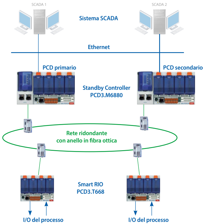
Topologia di rete raccomandata con reti fisicamente separate e anello in fibra ottica
