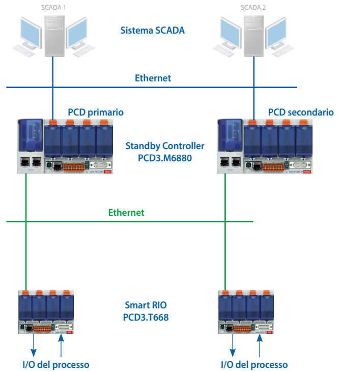
Reti fisicamente separate in una topologia a stella con componenti standard
