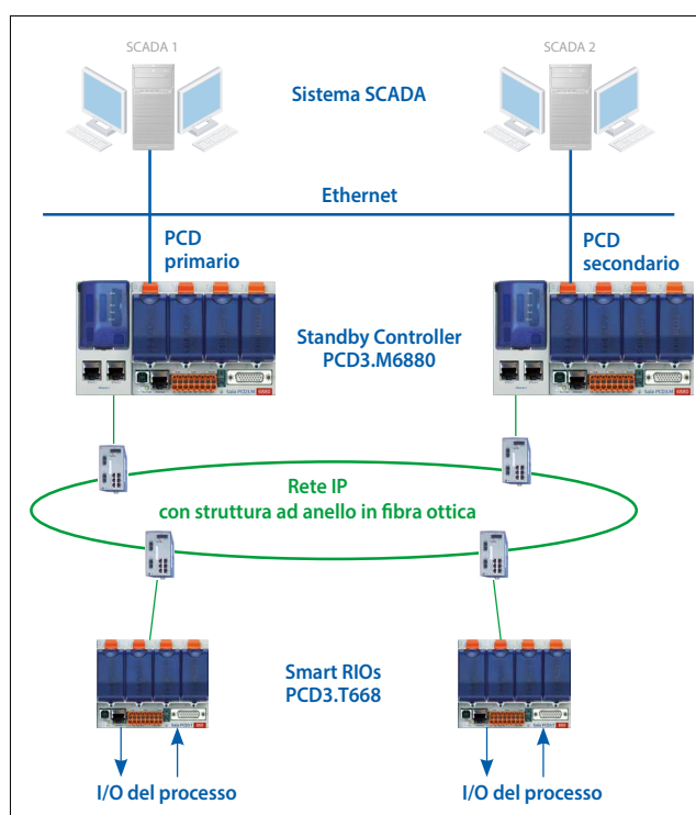
Tipica struttura di un sistema ridondante con due Standby Controller PCD3.M6880 e Ethernet Smart RIO PCD3.T668.
