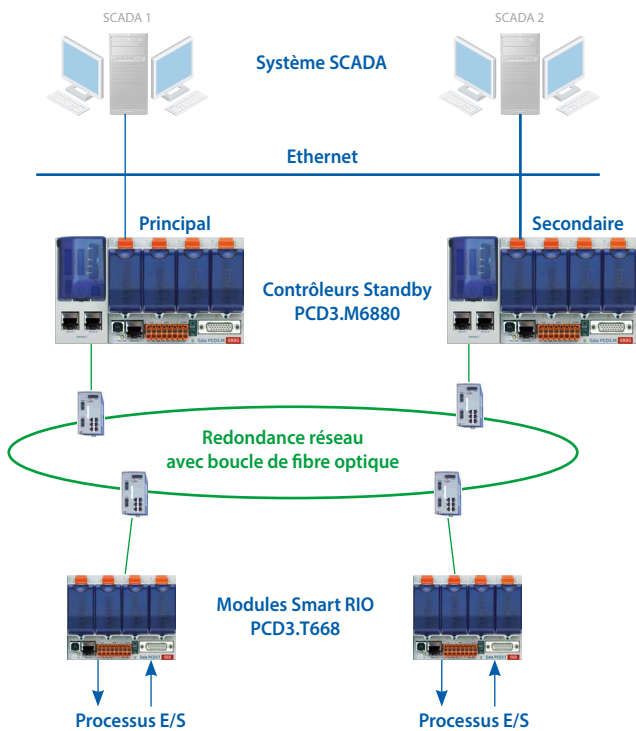
Topologie réseau recommandée avec des réseaux physiquement séparés et un boucle de fibre optique
