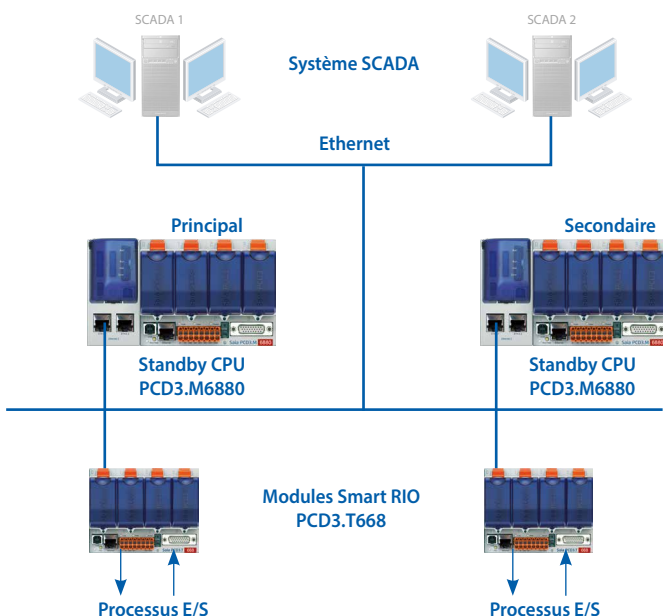
Réseau physique partagé dans une topologie en étoile avec des composants standard
