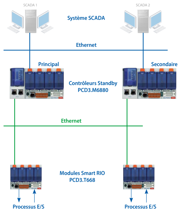
Réseaux physiquement séparés dans une topologie en étoile avec des composants standard
