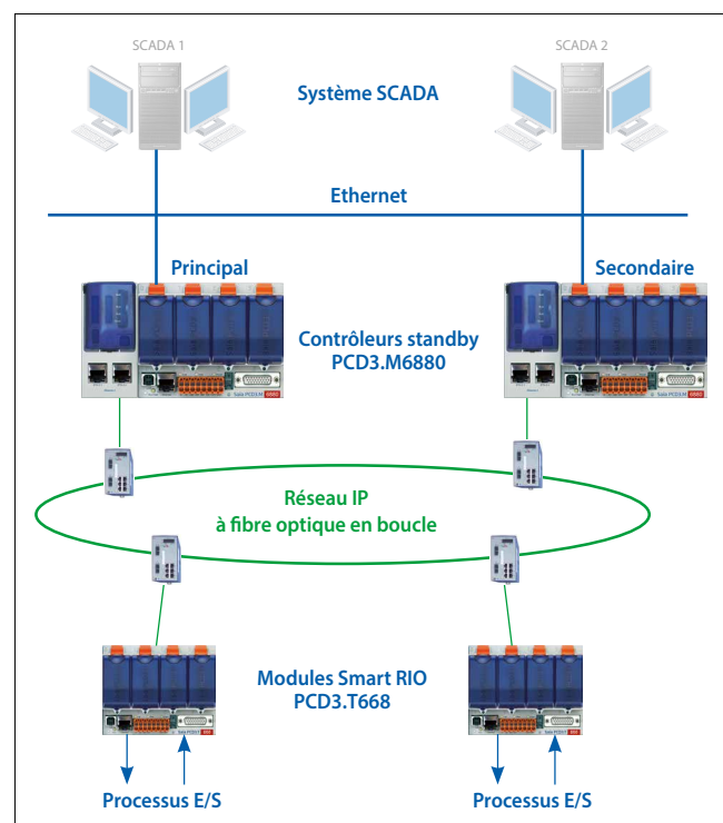
Disposition typique d'un système de redondance avec deux appareils de secours PCD3.M6880 et des modules Smart RIO Ethernet PCD3.T668.
