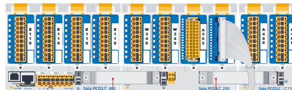
Connettore di espansione PCD3.K010
