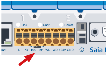
Anschlussklemme 3 und 4 für Interrupt-Eingänge Int0 und Int1
