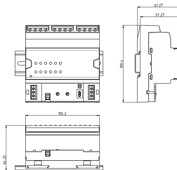
Largeur du boîtier 6 UD (105 mm) Compatible avec les armoires électriques (selon DIN 43880, dimensions 2 x 55 mm)
